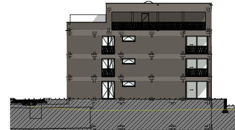
Ansicht Nord-West
