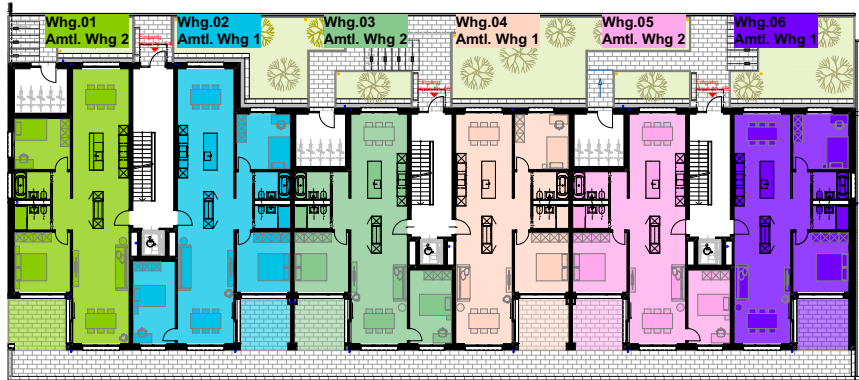
Grundriss Erdgeschoss
