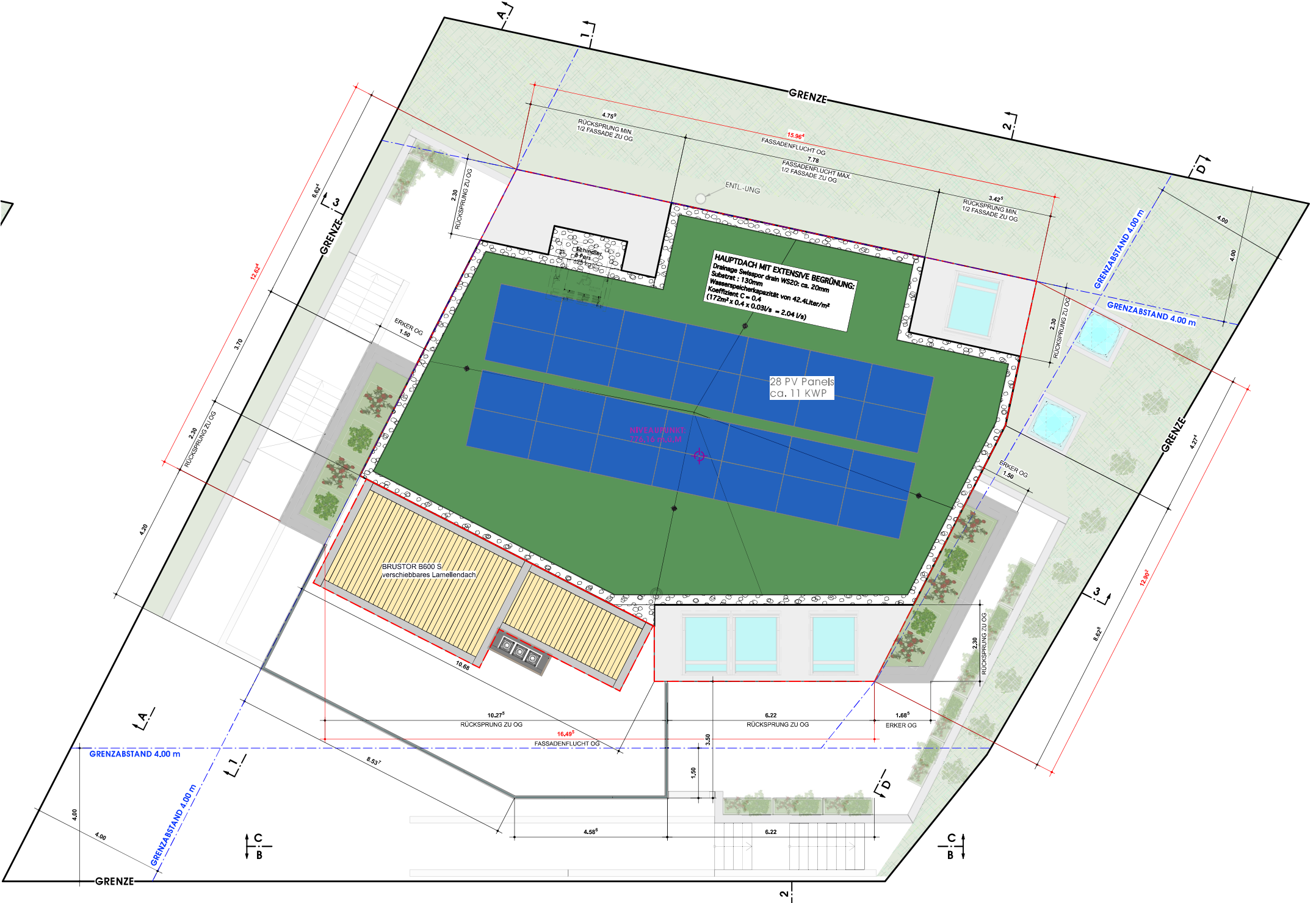
DACHAUFSICHT
